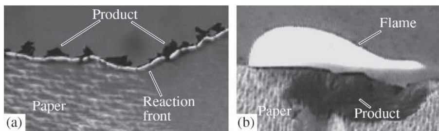
Рис. 4. Режимы горения: (а) режим медленного распространения пламени и (b) режим быстрого распространения пламени [10].
