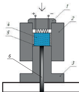
Рис. 6. Схема СВС-экструзии: 1 – иницилирующее устройство, 2,3- элементы пресс-формы, 4 – исходная шихтовая заготовка, 5 – теплоизоляционная оболочка, 6 – экструдированный стержень.
