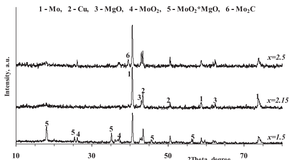
Рис. 9. Диффрактограммы продуктов сгорания смесей \text{MoO}_3 + \text{CuO} + 1.2\text{Mg} + x\text{C} .
