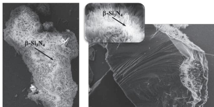
Рис. 4. Образование вискерсов \beta\text{-Si}_3\text{N}_4 в порах частиц кремния: а – в реакционных порах частицы кремния («темплатный» тип), б – на границе раздела твердое-газ («взаимоориентированные»).
