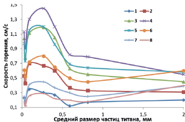
Рис. 13. Влияние дисперсности порошка Ti на скорость горения смеси с ферробором. T_0 = 500^\circ \text{C} . \text{Ti}/\text{B}_{\text{ат}} : 1 – 0,35, 2 – 0,45, 3 – 0,70, 4 – 0,86, 5 – 1,05, 6 – 1,57, 7 – 2,44, 8 – 2,78.
