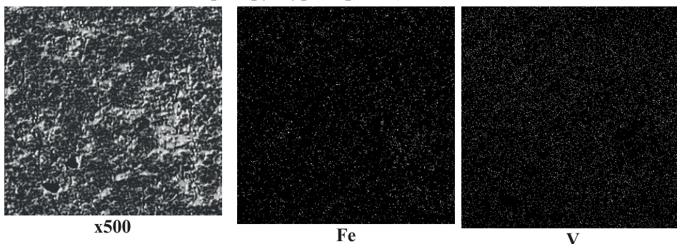
Рис. 4. Микроструктура и микроанализ продуктов горения \sigma -(Fe-V).
