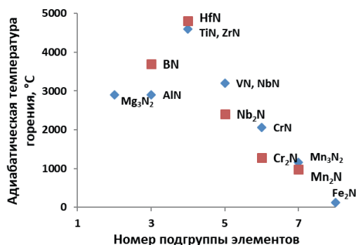
Рис. 2 Адiabатическая температура горения нитридов.
