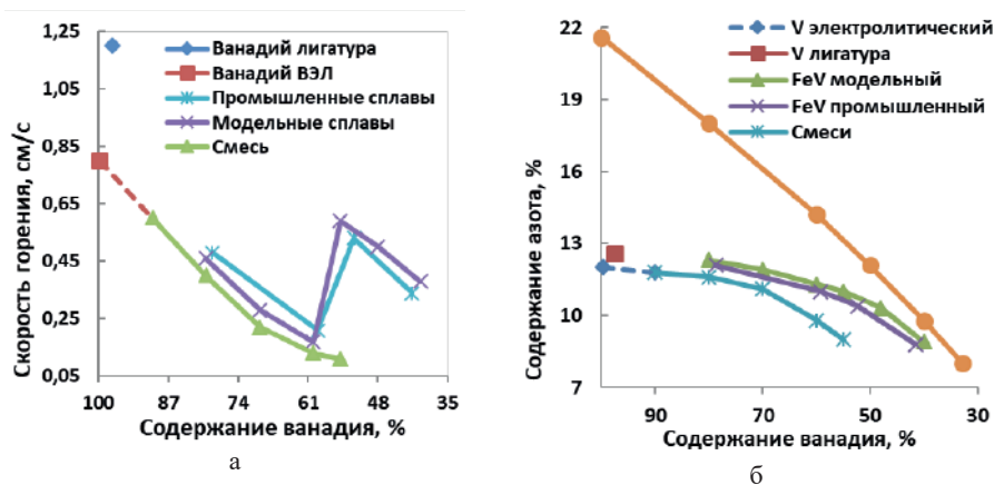
Рис. 3. Влияние концентрации ванадия на скорость горения феррованадия (а) и содержание азота в феррованадии (б).
