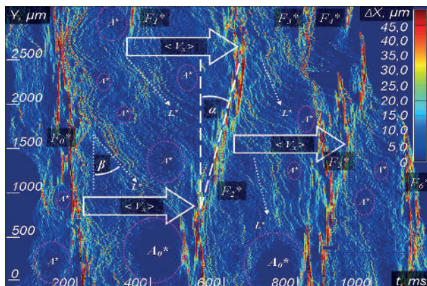
Рис. 16. Пример карты ДХС неустойчивого режима горения: поле мгновенных скоростей теплопереноса V(x,y) = \Delta X / \Delta t в волне СВС: F_i^* - дискретный фронт тепловыделения; L_i^* - линии эстафетного горения; A_i^* - ареал диффузионного выравнивания; \sin(\alpha)F_i^* и \sin(\beta)L_i^* - нарушение когерентности волны (время и пространство локализации).
