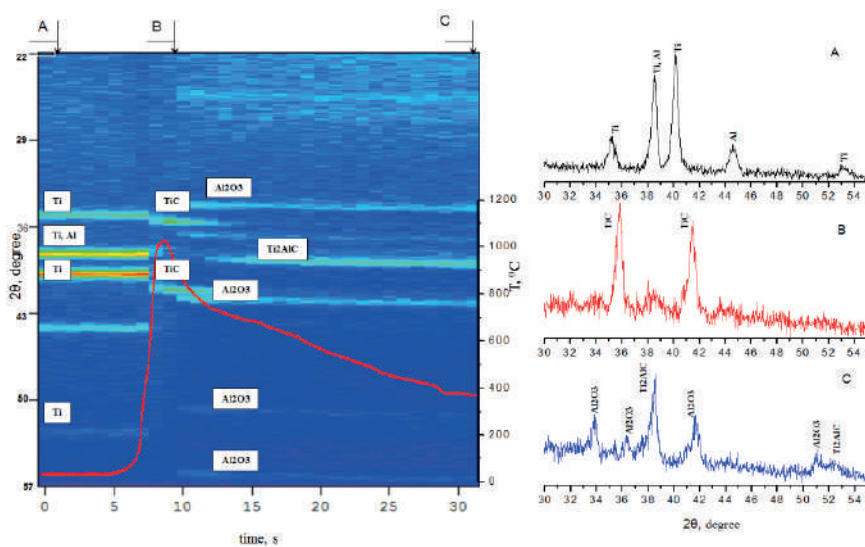
Рис. 16. Дифракционная картина горения смеси 3Ti-2Al-C на воздухе.
