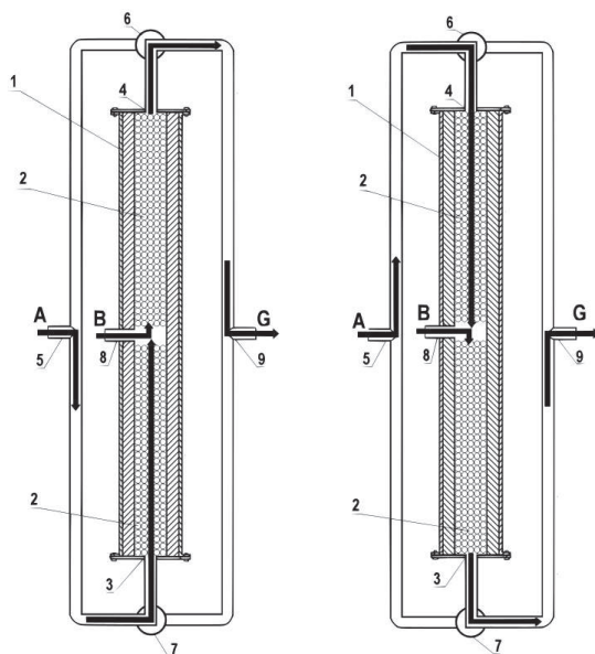
Рис. 2. Реактор с обратимым потоком заполненный пористой матрицей (схема). 1 – реактор, 2 – пористая матрица, 3 и 4 – вводы, 5 – коллектор реагирующего газа, 6 и 7 –трёхходовые краны, 8 – коллектор газообразных продуктов. Слева – потоки в первом полуцикле, справа – во втором.
