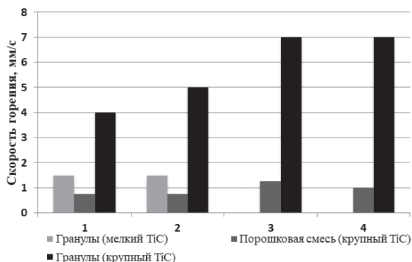
Рис. 15. Скорости горения порошковой и гранулированной смеси TiC+Ti в потоке азота при различных условиях проведения экспериментов: 1 – 2 атм. сверху, 1 атм. снизу; 2 – 2 атм. сверху, 1 атм. снизу + экран; 3 – 2 атм. сверху, 0 атм. снизу (вакуумный насос); 4 – 2 атм. сверху, 0 атм. снизу (вакуумный насос) + экран.
