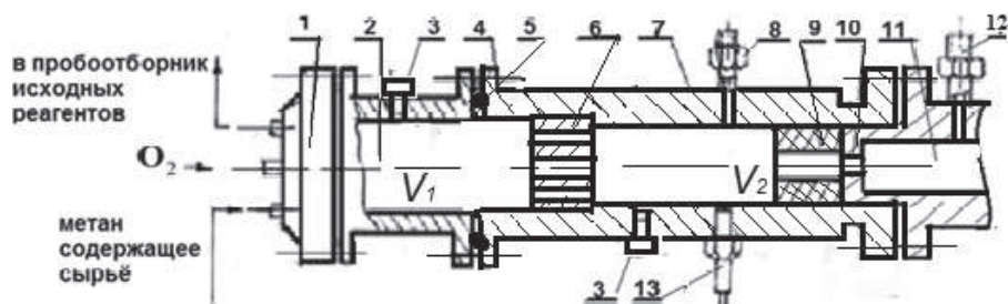
Рис. 2. Общая блок-схема для сборки различных компоновок конструкции РХПТ. 1 – центробежная форсуночная головка от ЖРД МДТО-123; 2 – камера турбулентного смешения; 3 – датчик давления; 4 – крепёжные болты; 5 – уплотнительное алюминиевое кольцо; 6 – турбулизатор; 7 – корпус камеры сгорания; 8 – штуцер для подачи дополнительного кислорода при поджиге; 9 – керамическая вставка; 10 – выходное критическое сечение камеры сгорания; 11 – камера для отбора проб продуктов сгорания; 12 – штуцер для отбора проб продуктов сгорания; 13 – свеча зажигания.
