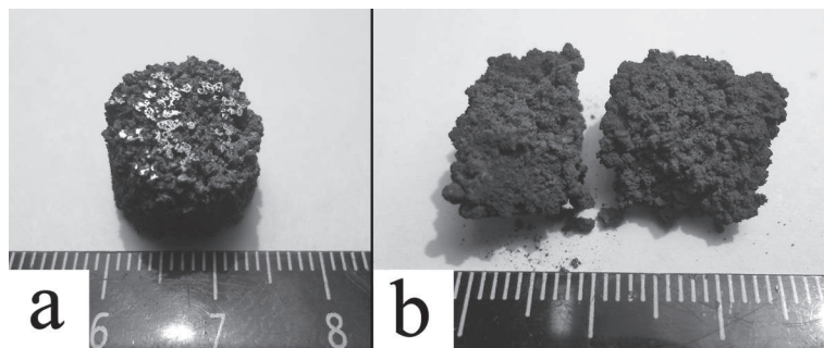
Рис. 19. Поперечный срез (а) и излом (б) продукта синтеза гранул Ti+C+25\%Ni в потоке газа: а - в потоке аргона, б - в потоке азота. (Перепад давлений 1 атм.).
