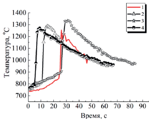
Рис. 4. Термограммы горения для системы (SiO 2 + 37,5%Al) с не активированным кварцем (1) и после МХО в течение 10 (2), 20 (3) и 30 (4) мин.
