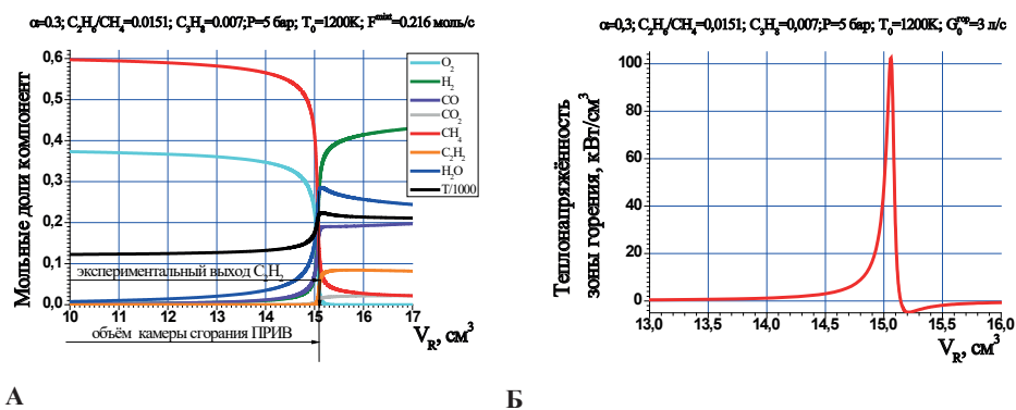
Рис.15. Численное моделирование процесса окисипиролиза ПГ зимнего состава с кислородом по мере прохождения газовым потоком объёма камеры сгорания V_{\text{R}} в модели ПРИВ. Зависимости: А - концентраций реагентов, продуктов и T_{\text{прод}} ; Б – максимальной теплонапряжённости зоны горения.
