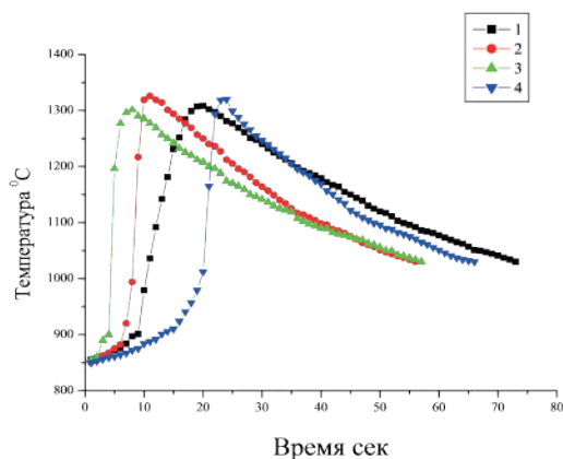
Рис. 9. Термограммы горения системы [(SiO 2 + 37,3%Al)] с 5% волластонита FW100, активированного в течение 10 мин. с кремневой (1) и янтарной кислотой (2), с поливинилловым спиртом (3) и без модификатора (4).
