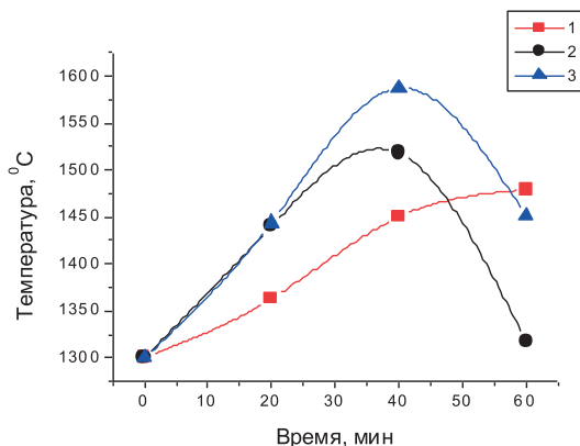
Рис. 18. Зависимость максимальной температуры горения СВС-образцов с 10 % волластонита после УЗ-обработки в воде от времени при частоте 40 (1), 100 (2) и одновременном воздействии 40 и 100 кГц (3).
