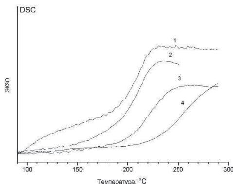
Рис. 9. Тепловыделение в образцах состава 3\text{Ni} + \text{Al} (3 мин МА) без предварительного отжига (1) и отожженных при температурах 150 (2), 210 (3) и 250°C (4).
