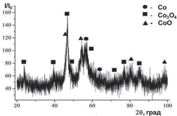
Рис. 31. Спектр РФА катализатора 95Co-5Ce.
