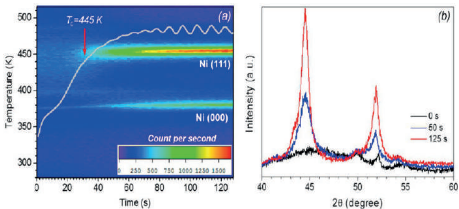
Рис. 20. Дифракционная картина кристаллизации аморфного Ni.
