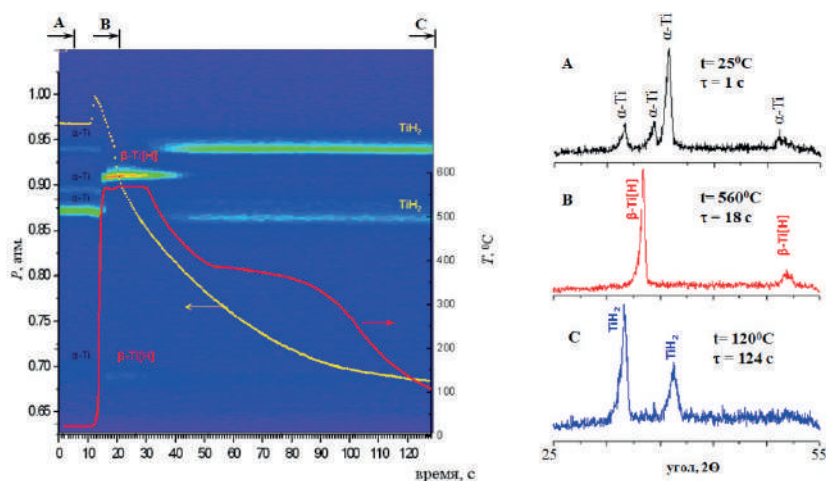
Рис. 6. Дифракционная картина гидрирования Тi.
