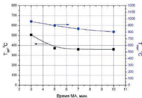
Рис. 4. Зависимости температуры инициирования и максимальной температуры теплового взрыва состава Ti + 4 мас. % C от времени предварительной МА.
