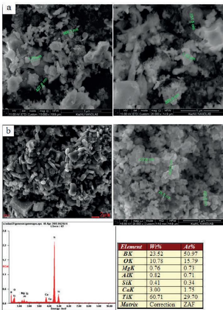
Рис. 4. Микроструктура продуктов СВС и элементный анализ (SEM) системы TiO_2 - B_2O_3 (руда) – Mg (а–без МА, б– 5 мин МА).
