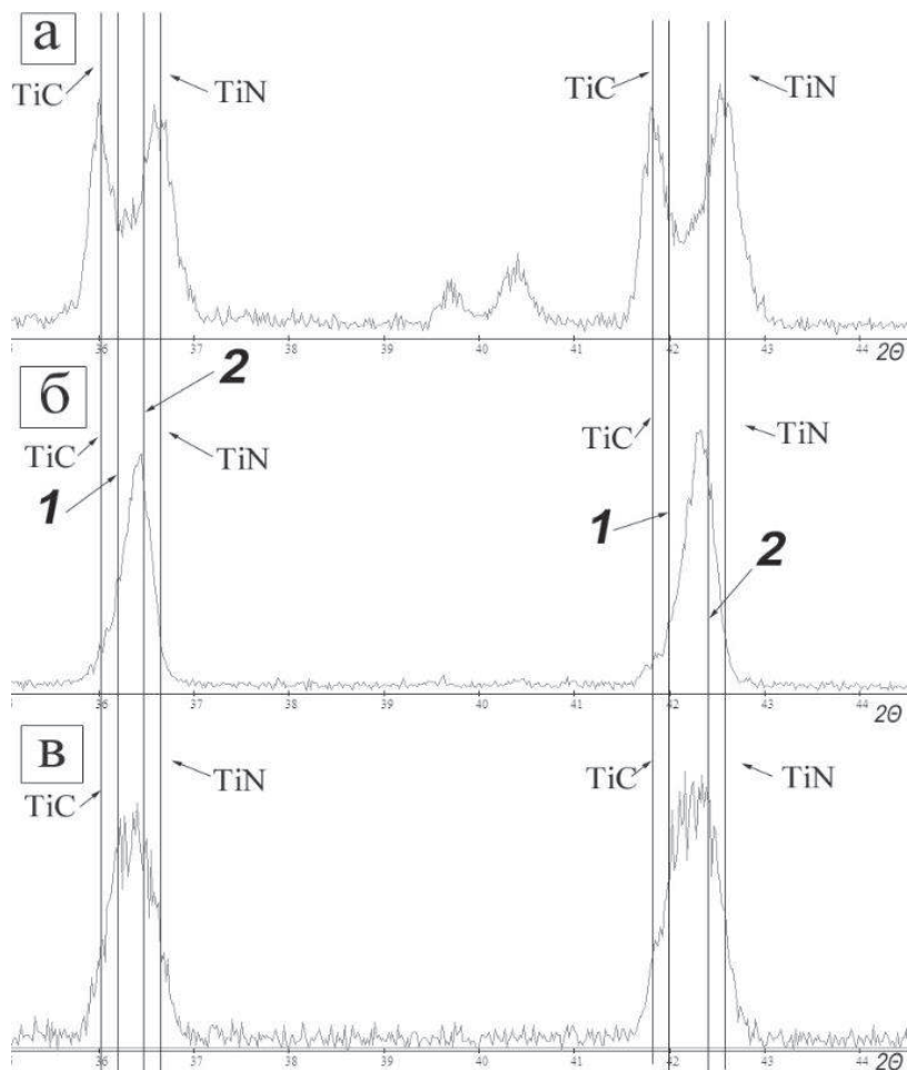
Рис. 16. Рентгенограммы главных пиков продуктов горения: а – порошковой смеси из крупного TiC, б – гранулированной смеси из крупного TiC, в - гранулированной смеси из мелкого TiC; линии 1 соответствуют максимумам двух первых пиков карбонитрида титана состава TiC_{0.7}N_{0.3} (карточка 42-1489), а линии 2 - TiC_{0.3}N_{0.7} (карточка 42-1488).
